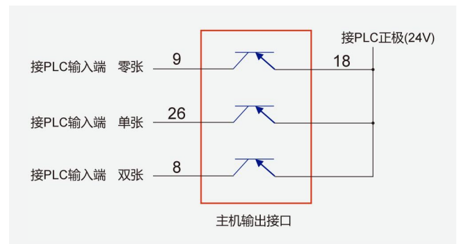
图 2-7: 主机输出接口与 PLC 接线图
