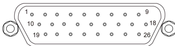
图 2-6: 输入输出接口示意图
