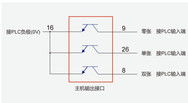
图 2-7: 主机输出接口与 PLC 接线图
