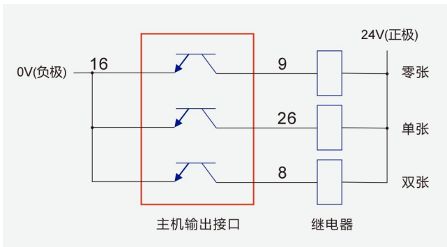
图 2-6: 主机输出接口与继电器接线图
