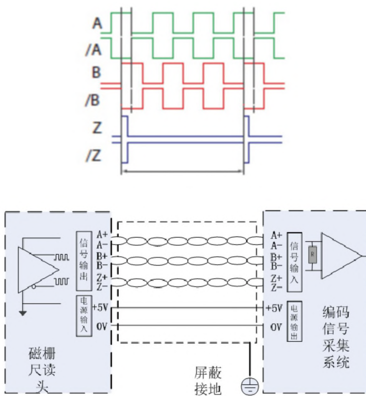
图 1-2: 输出信号
